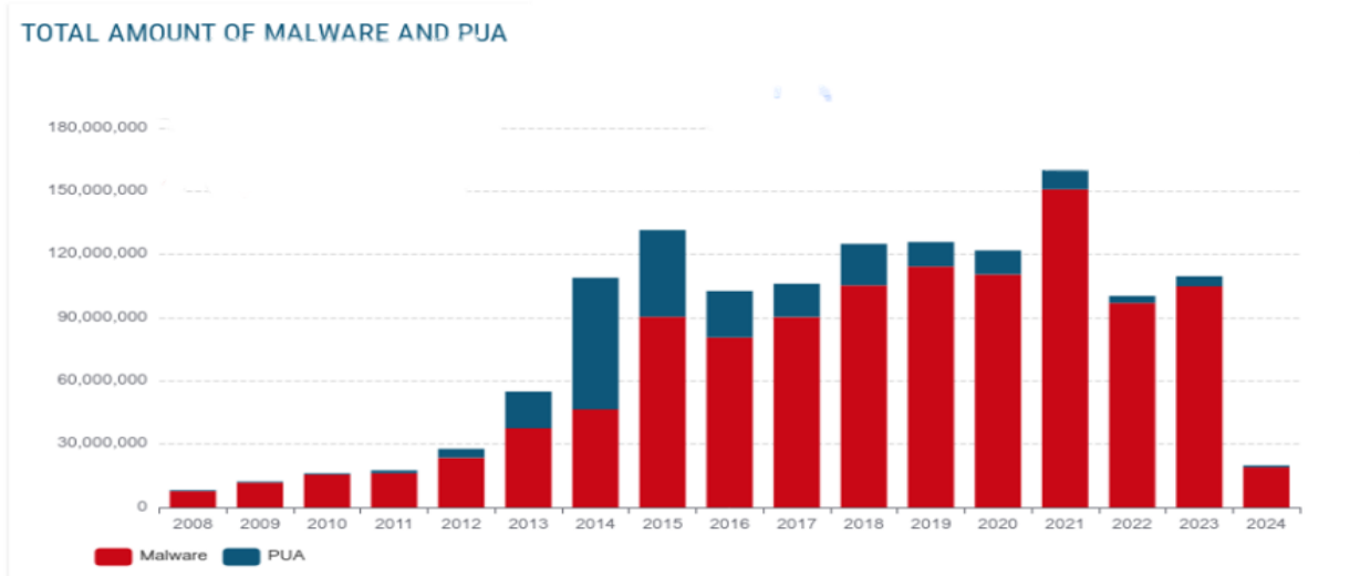
Fig.5. New Malware
