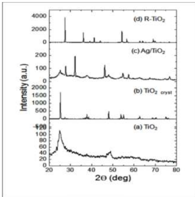
Fig. 6. XRD pattern for (a) \text{TiO}_2 (b) \text{TiO}_2 cryst (c) \text{Ag}/\text{TiO}_2 (d) \text{R-TiO}_2 .
