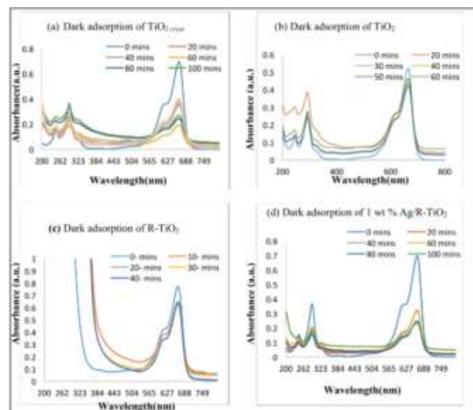
Fig. 7. Dark absorption of (a) \text{TiO}_2 cryst (b) \text{TiO}_2 (c) \text{R-TiO}_2 and (d) 1 wt% \text{Ag}/\text{R-TiO}_2 .
