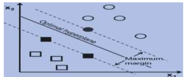
Fig.1. SVM
