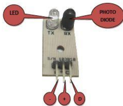
Fig. 3. IR Sensor
