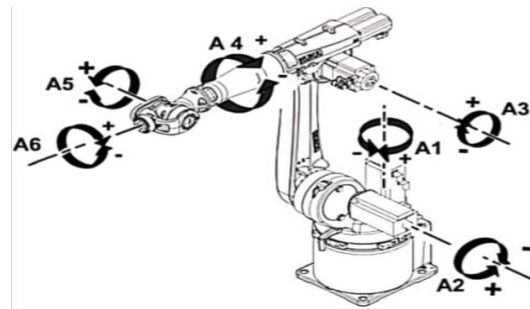
Fig. 4. Kuka Robot
