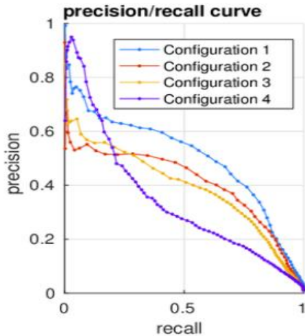
Fig.18. Precision/Recall curve.
