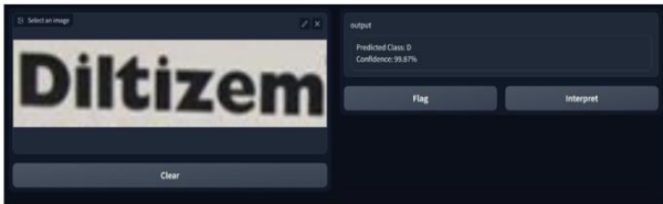
Fig. 16. Gradio output-D
