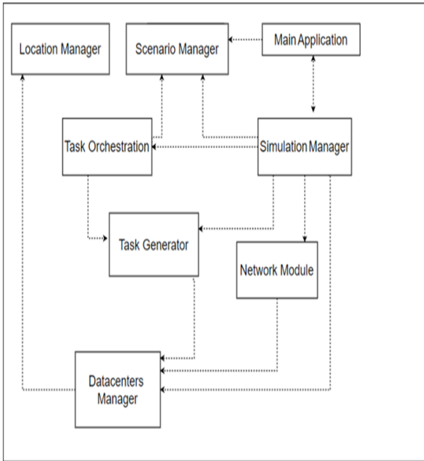
Figure 2. PureEdgeSim Module
