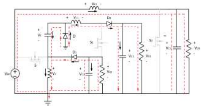
Fig.4:Mode2
